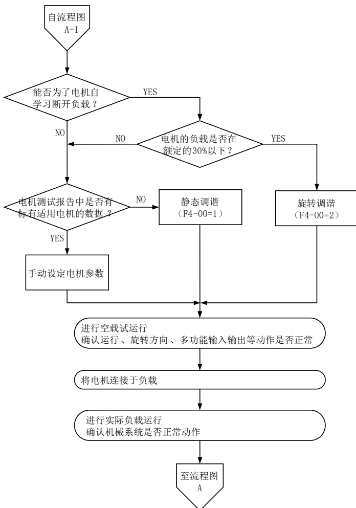
图 4-6. 闭环矢量控制方式运行步骤
