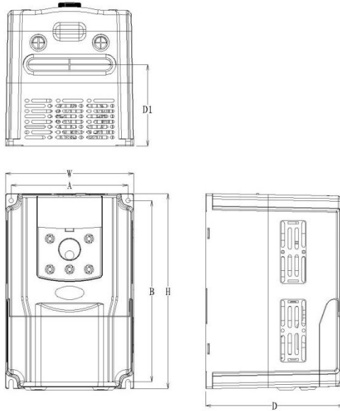
图 2-4 塑壳变频器外型尺寸及安装尺寸示意图
