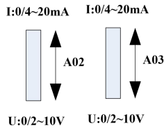
附录B：图7 CM580IO2拨码开关切换图
