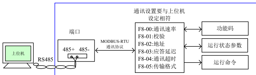
图4-30. 通讯设置示意图
