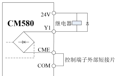
内部供电接线图
