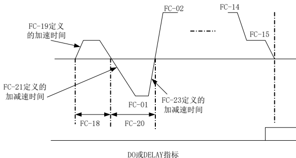
图5-28. 简易PLC示意图
