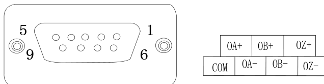
附录 B: 图 11 CM580PG4 端子图
