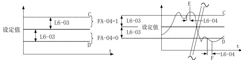
图5-32. 唤醒示意图
