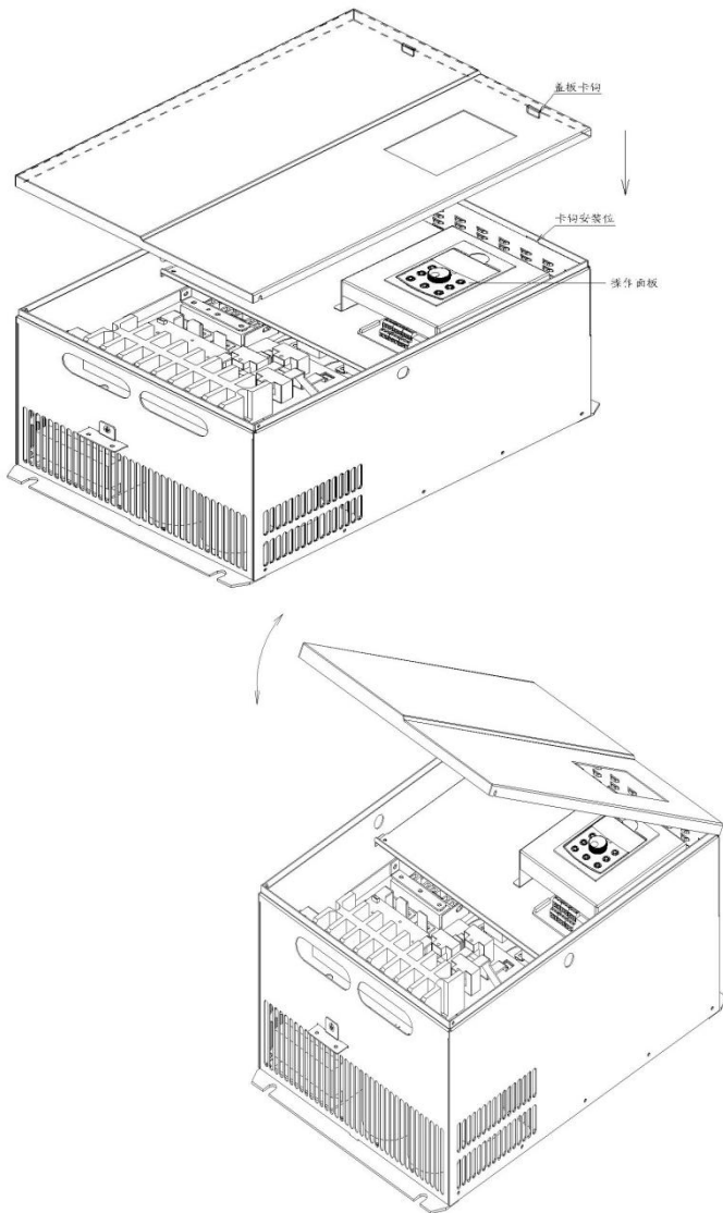
图 3-3 钣金外壳下盖板拆卸图
