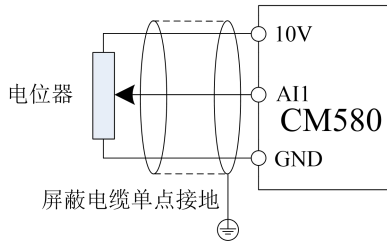
图 3-7 模拟量输入端子接线示意图
