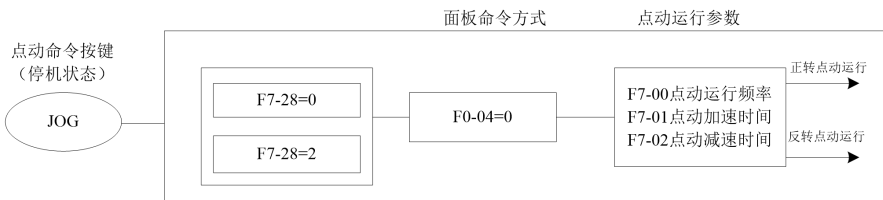
图4-15. 点动参数设定示意图
