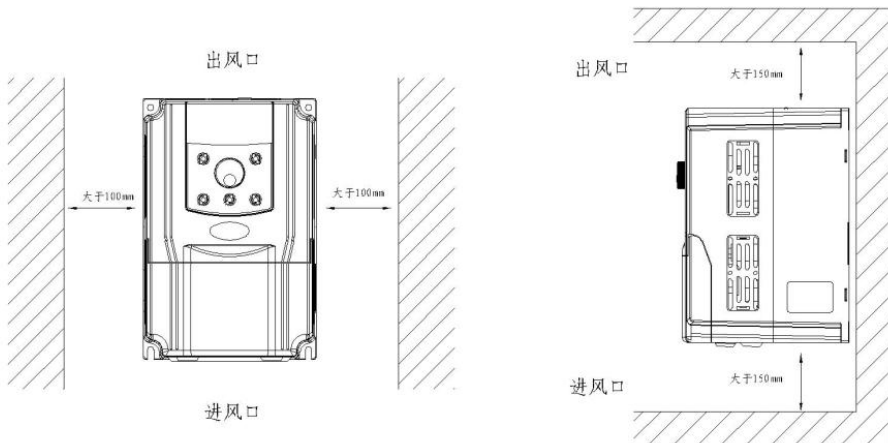
单体安装图
