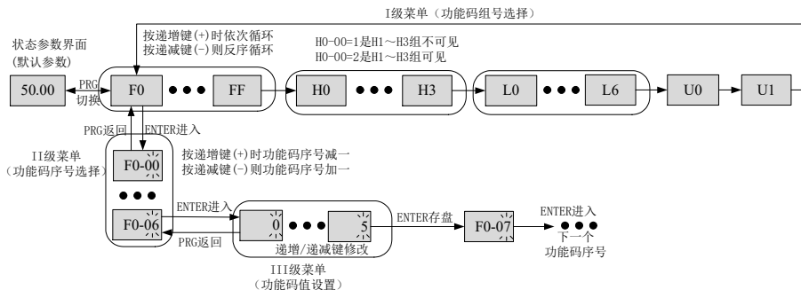
图 4-2 三级菜单操作流程图
