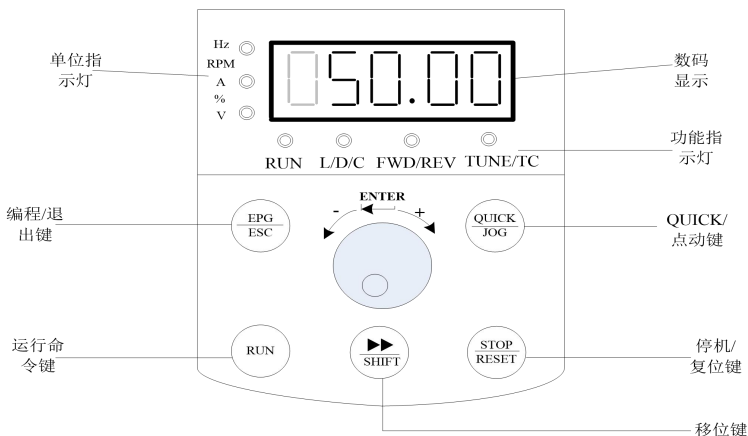
图 4-1 操作面板示意图 1(标准配置 LED 键盘 1)
