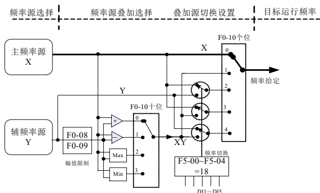
图5-1. 频率源叠加示意图
