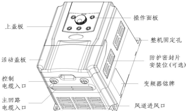
图 2-3 变频器外型图
