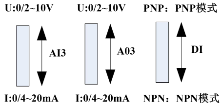
附录 B: 图 3CM580I01 拨码开关切换图
