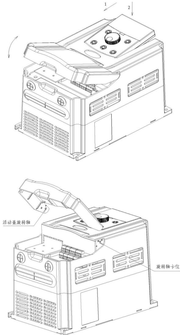
图 3-2 塑胶外壳下盖板拆卸图
