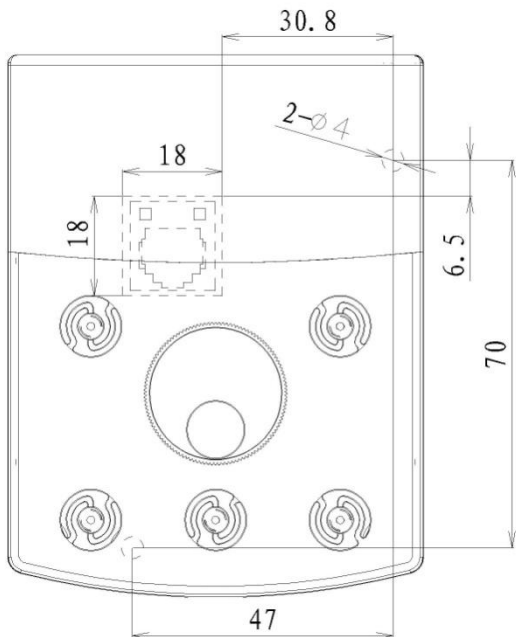
图 2-7 外引键盘不带托盘安装开孔示意图
