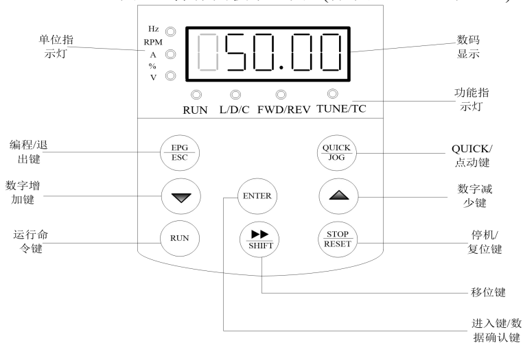
图 4-1 操作面板示意图 1(标准配置 LED 键盘 1)
