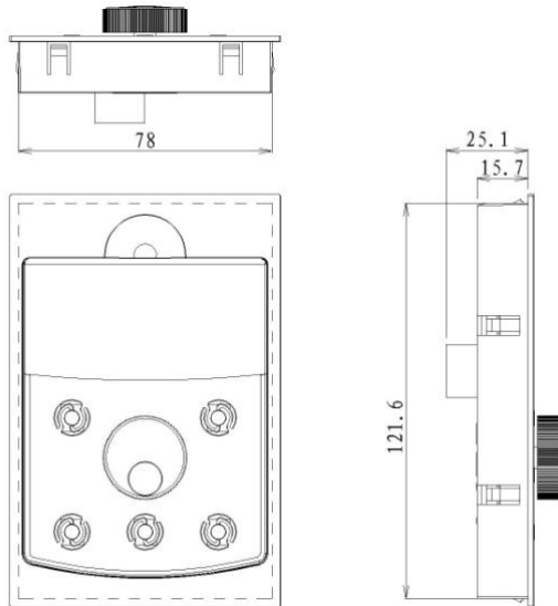
图 2-6 外引键盘带托盘安装尺寸示意图
