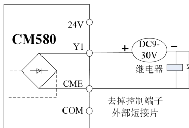
外部供电接线图
