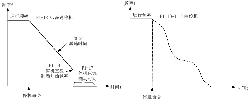
图4-13. 停机示意图
