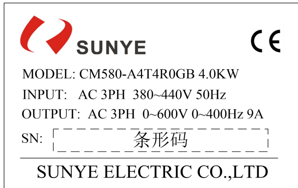
图 2-2 铭牌
