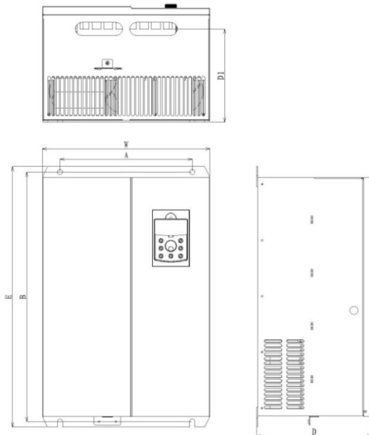
图 2-5 钣金件变频器外型尺寸及安装尺寸示意图
