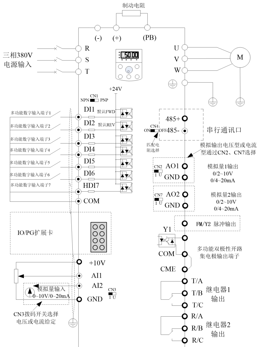
图 3-4 30kW 以下内置制动单元三相变频器
