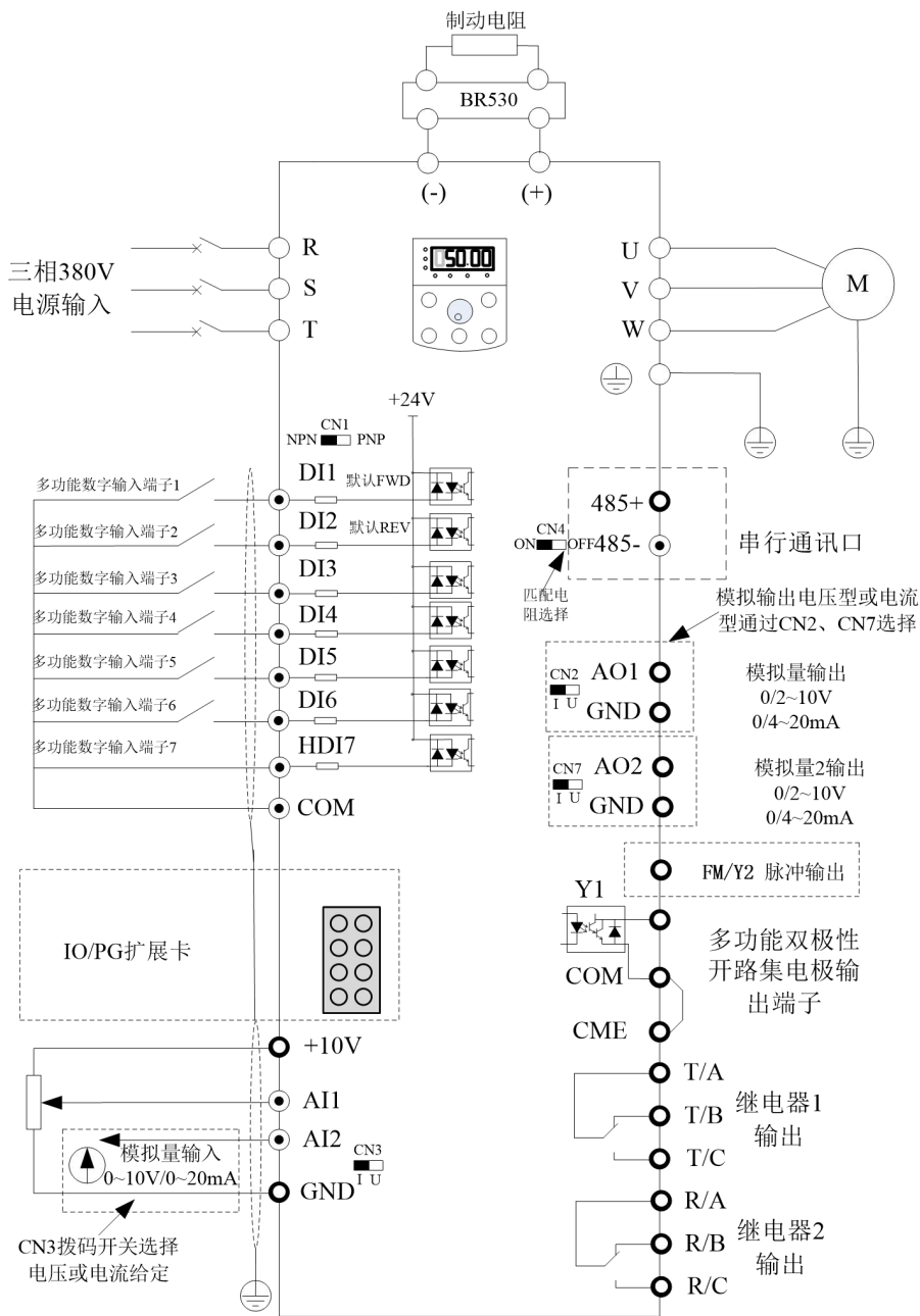
图 3-5 37kW ~ 55kW 三相变频器
