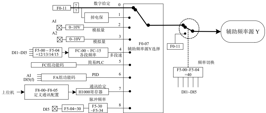
图4-18. 主频率源设置示意图
