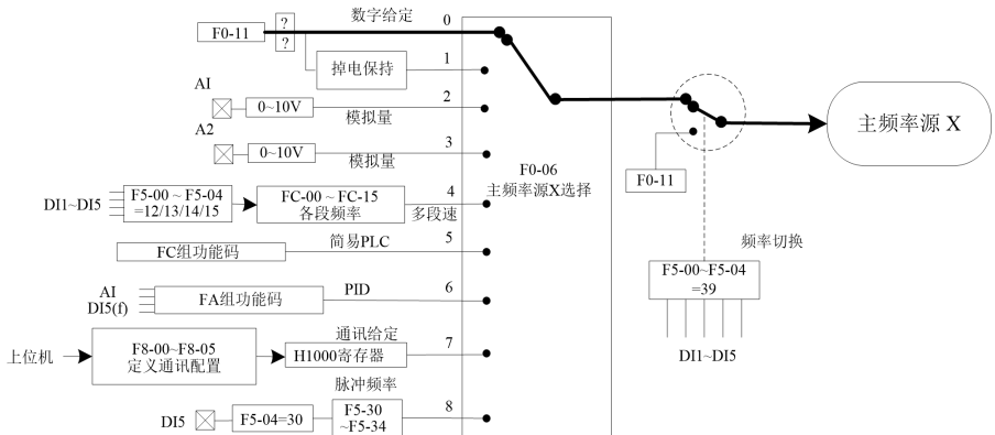
图4-17. 主频率源设置示意图
