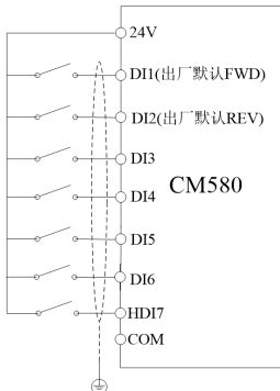
图3-8 四种不同模式下数字输入端子接线图
