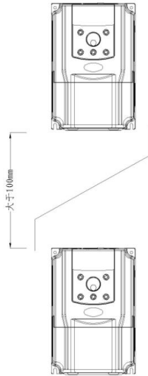
图 3-1CM580 变频器安装示意图
